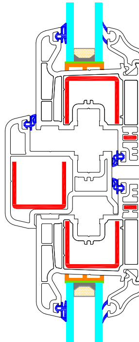
A-2 Detail
