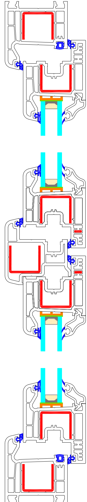
A-1 DETAYI
