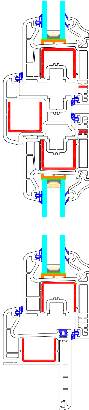
A-2 DETAYI
