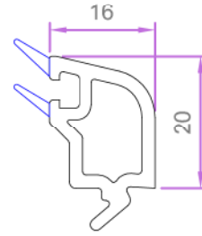
OVAL Ç.CAM ÇİTASI 24mm
