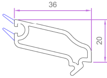
TEK CAM ÇİTASI - 4mm
