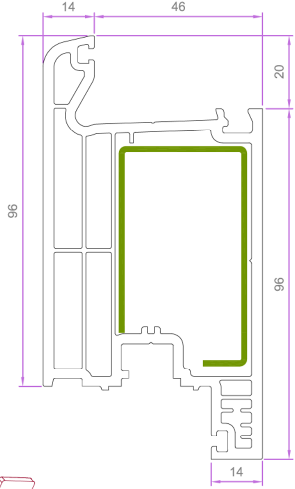
AB 01009 3308 ALÜMİNYUM EŞİK PROFİLİ
