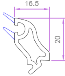
ÇİFT CAM ÇİTASI 24mm
